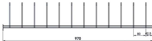
RZUT
