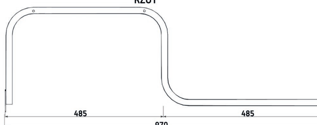
RZUT
