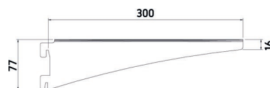
RZUT
