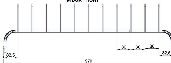
WIDOK FRONT
