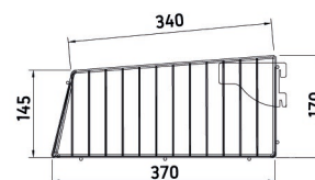
WIDOK BOK
