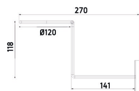
WIDOK BOK
