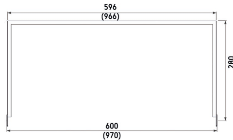
RZUT
