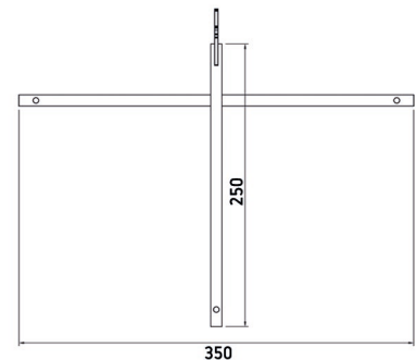
WIDOK BOK
