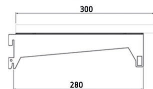
WIDOK BOK
