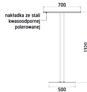
WIDOK BOK
