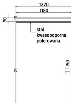
WIDOK FRONT
